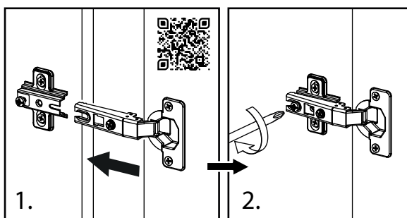
Петля без доводчика
