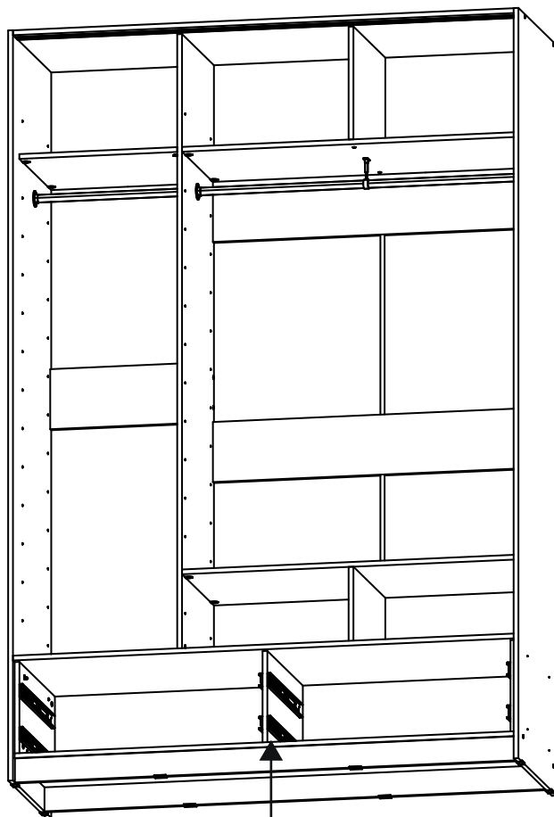
Шариковые направляющие ↓
