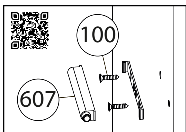
Петля с доводчиком
